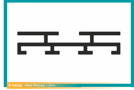
TEKNİK DETAY -TECHNICAL DETAIL
