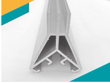
A KESİT -SECTION
